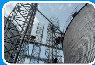
JASA INSTALASI TOWER DAN SILO Buduran Sidoarjo 22 Februari 2025
